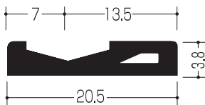
納まり図
